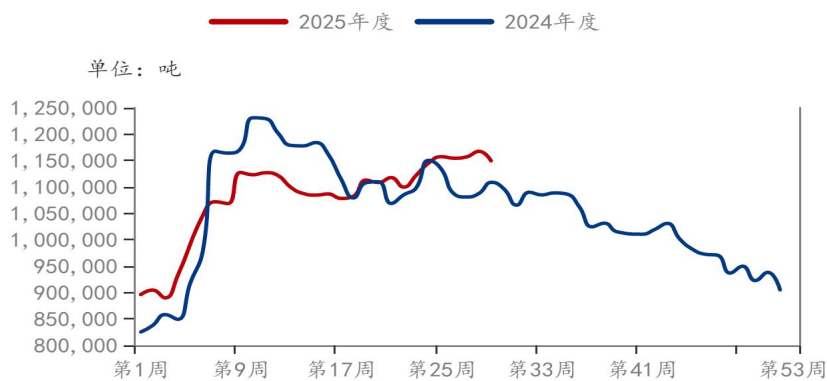
不锈钢：89家样本企业：库存：中国（周）
